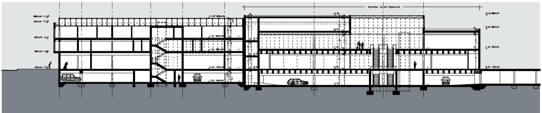
Schnitt B-B
