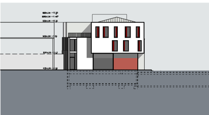
Seitenansicht
